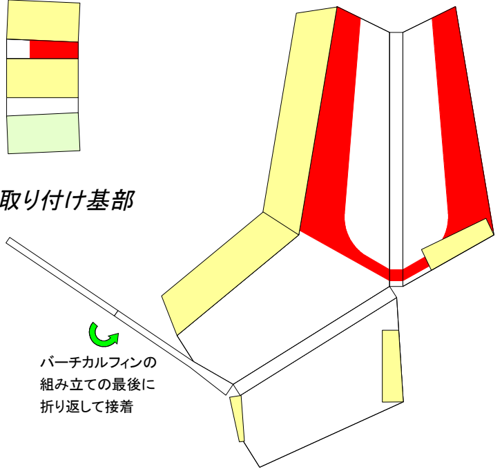
バーチカルフィン
